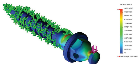
Figura 7 - Análise de elementos finitos em parafuso ortodôntico.
