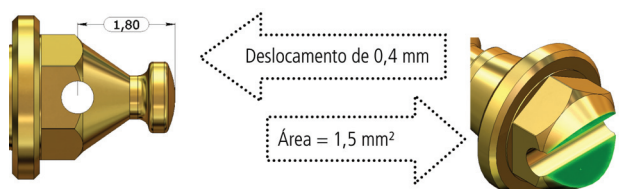
Figura 6 - Modelo de parafuso ortodôntico com recuo de 0,4 mm em relação ao modelo original e representação da área da seção resistente no ponto mais crítico.
