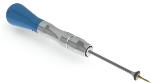
Figura 1 - Montagem da chave de inserção com parafuso ortodôntico.
