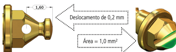
Figura 5 - Modelo de parafuso ortodôntico com recuo de 0,2 mm em relação ao modelo original e representação da área da seção resistente no ponto mais crítico.
