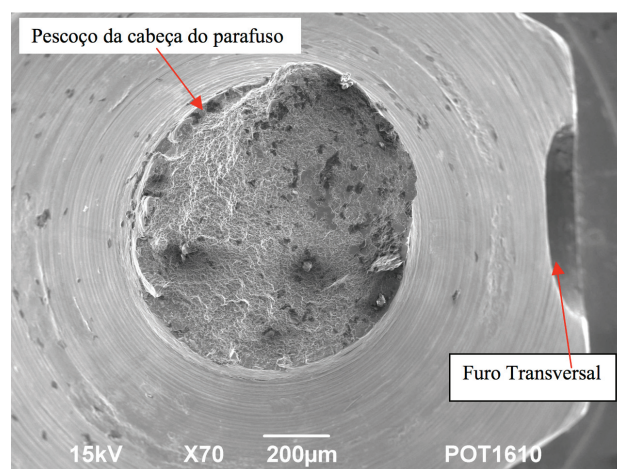
Figura 8 - Microscopia eletrônica de varredura de fratura após inserção do implante em resina.
