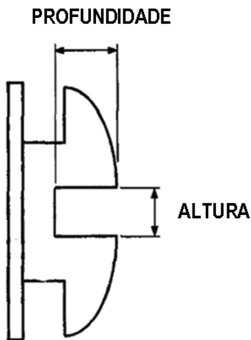
Figura 1 - Desenho esquemático do braquete com as medições da altura e profundidade efetuadas no microscópio óptico de medição universal
