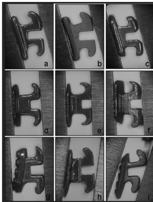
Figura 2 - Fotografias dos braquetes utilizados no estudo e posicionados no microscópio óptico de medição universal; a - Grupo 1 - aço inoxidável (Equilibrium 2°); b - Grupo 2 - titânio (Equilibrium ti°); c - Grupo 3 - cromo-cobalto (Topic°); d - Grupo 4 - aço inoxidável (Standard TP°); e - Grupo 5 - aço inoxidável (Serie light°); f - Grupo 6 - aço inoxidável (Kirium line°); g - Grupo 7 - aço inoxidável (Monobloc°); h - Grupo 8 - aço inoxidável (Convencional°); i - Grupo 9 - aço inoxidável (Monobloc Golden°).
