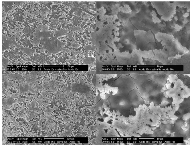
Figura 2. O recondicionamento por 10", do grupo decíduos, no esmalte condicionado por 15" e contaminado por 5" apresentou uma menor descaracterização da micromorfologia que a contaminação por 30".
