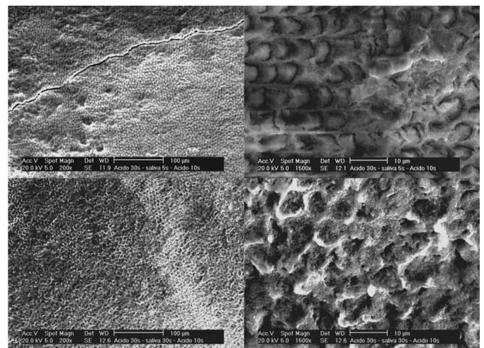
Figura 5. Não ocorreu um padrão de microporosidade aceitável no recondicionamento por 10" das amostras do grupo permanentes quando o esmalte condicionado previamente por 30" e contaminado por 5" ou 30".
