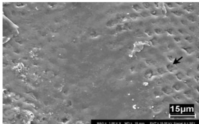
Figura 3. Experimental do Grupo 1, aumento no número e profundidade dos poros de desenvolvimento (1.000x).
