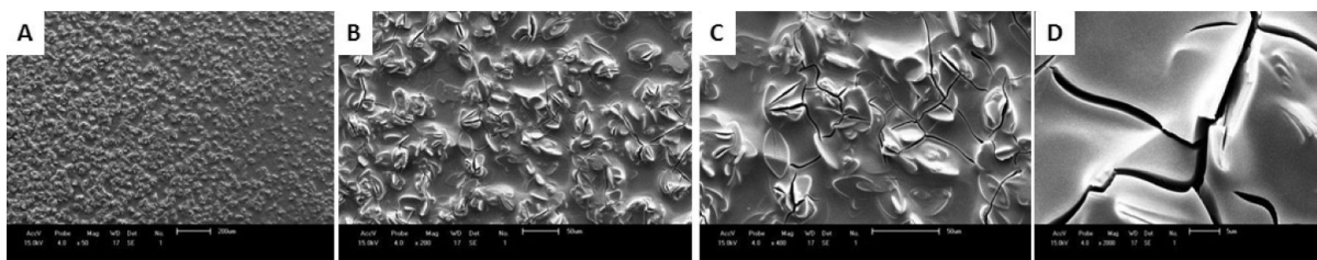
Figura 2 – Lamínula de vidro que ficou sete dias (amostra 1) em contato com o EDTA, com aumento de 50 (A), 200 (B), 400 (C) e 2.000 (D) vezes no MEV
