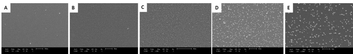
Figura 6 – Lamínula de vidro que permaneceu 24 horas (amostra 5, controle) em contato com a água destilada, com aumento de 100 (A), 200 (B), 400 (C), 1.000 (D) e 2.000 (E) vezes no MEV
