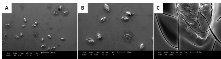
Figura 5 – Lamínula de vidro que ficou 30 minutos (amostra 4) em contato com o EDTA, com aumento de 50 (A), 100 (B) e 2.000 (C) vezes no MEV
