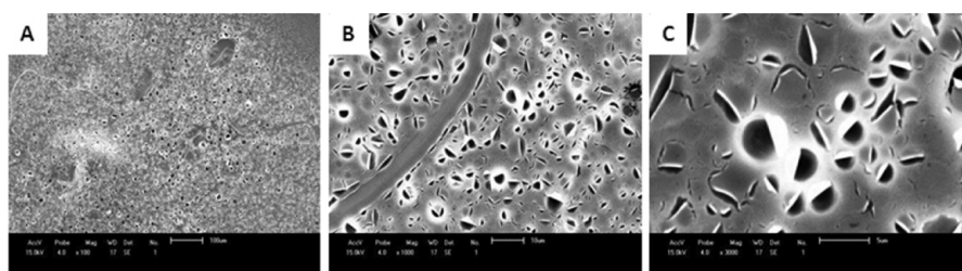
Figura 4 – Lamínula de vidro que esteve por 6 horas (amostra 3) em contato com o EDTA, com aumento de 100 (A), 1.000 (B) e 3.000 (C) vezes no MEV
